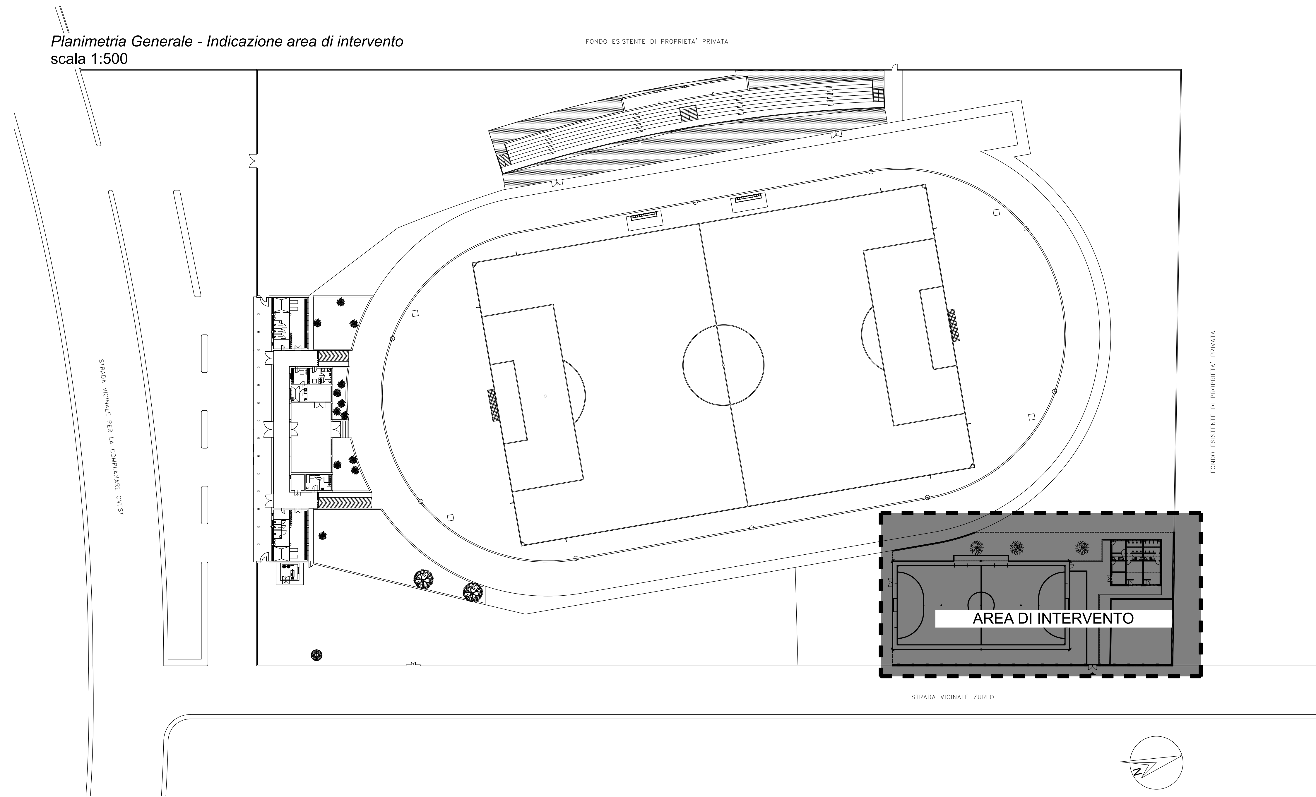
area di intervento _ segnature campi _ zone funzionali scala 1:100
